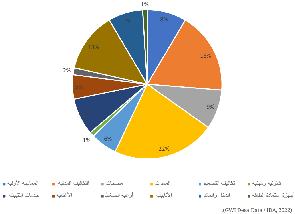
الشكل 7. تكلفة تحلية المياه بالتناضح العكسي التقليدي: تحليل الإنفاق الرأسمالي
