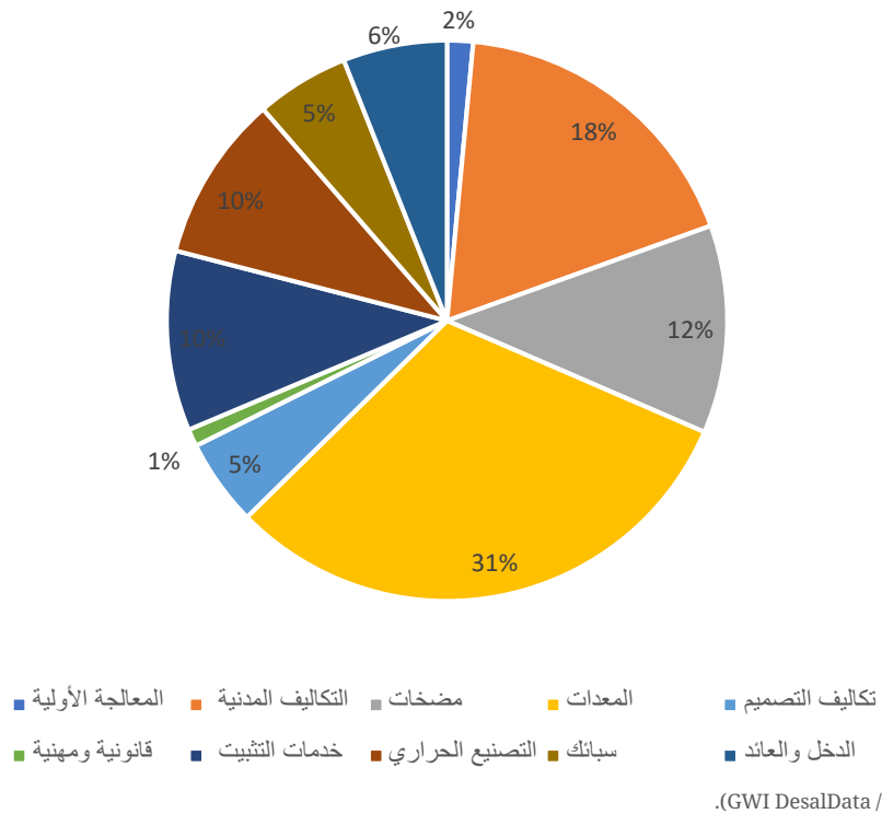
الشكل 8. تكلفة تحلية المياه في محطات التقطير الوميضي: تحليل الإنفاق الرأسمالي
